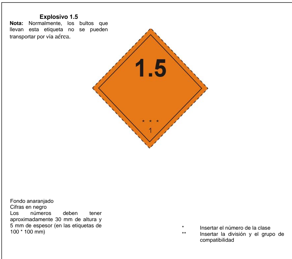
Figura. 5-4 Explosivo, Clase 1, División 1.5
